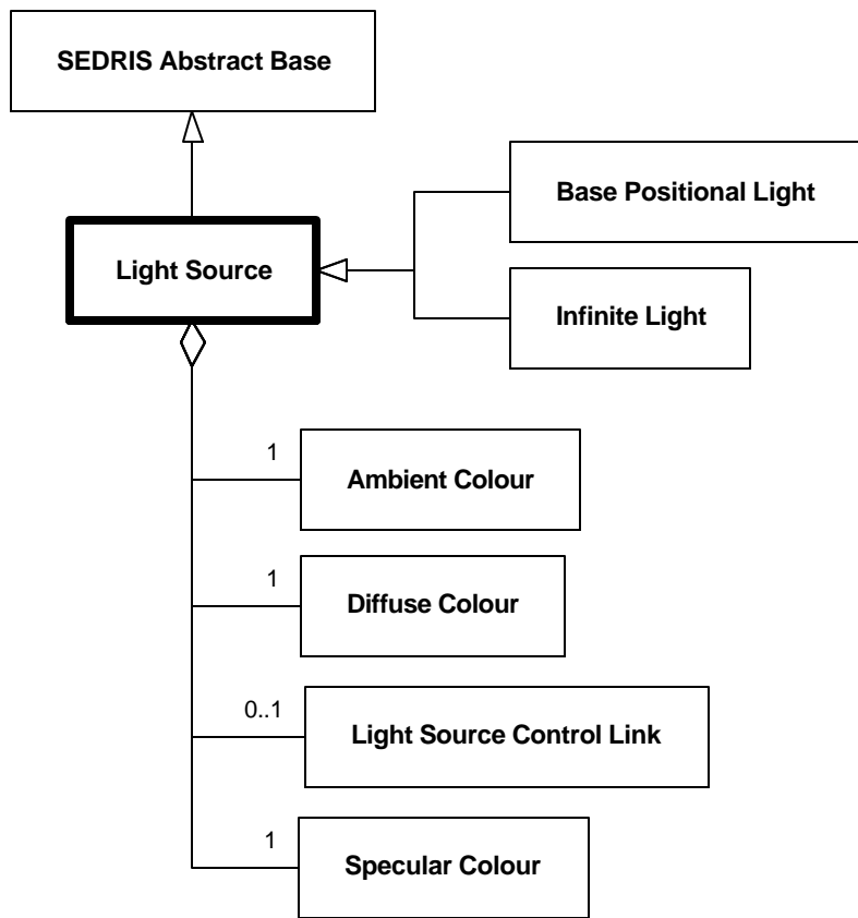
Diagram 6.156—DRM_Light_Source
