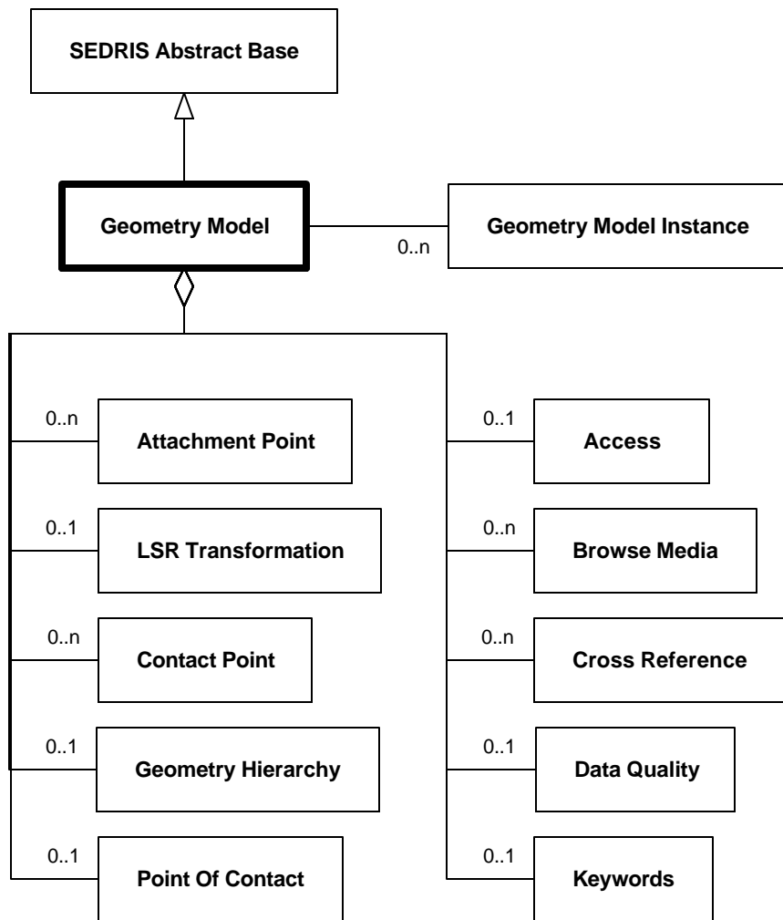
Diagram 6.118—DRM_Geometry_Model
