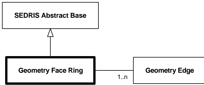
Diagram 6.114—DRM_Geometry_Face_Ring
