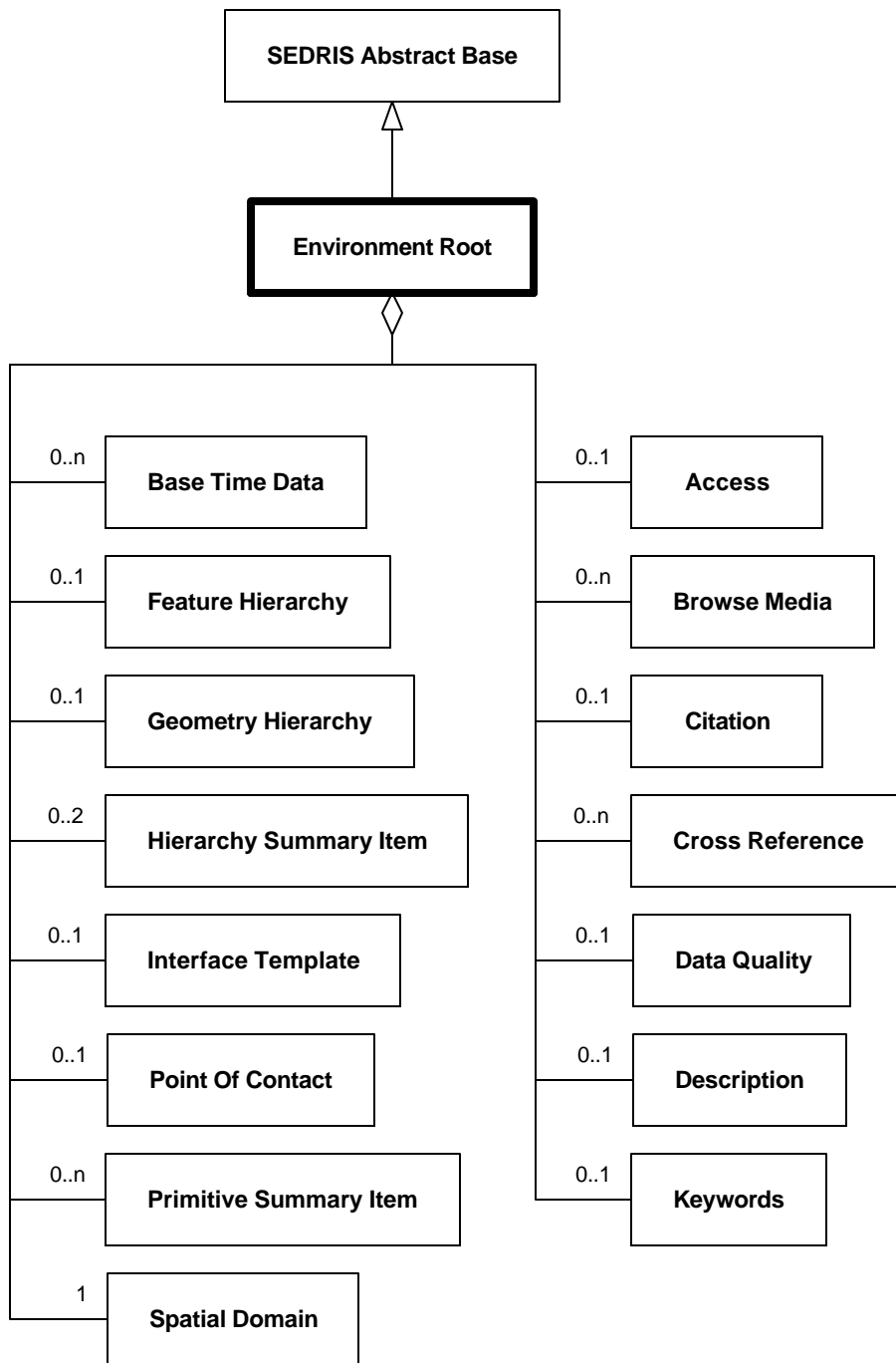
Diagram 6.84—DRM_Environment_Root
