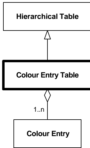
Diagram 6.52--DRM_Colour_Entry_Table
