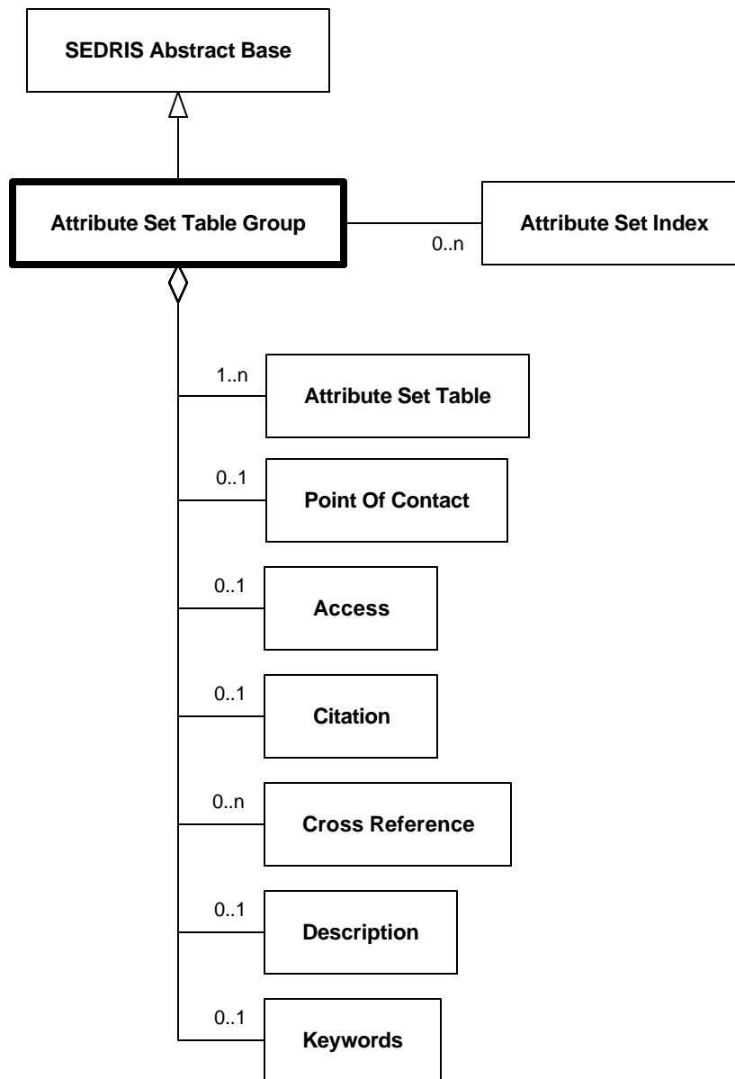
Diagram 6.24--DRM_Attribute_Set_Table_Group
